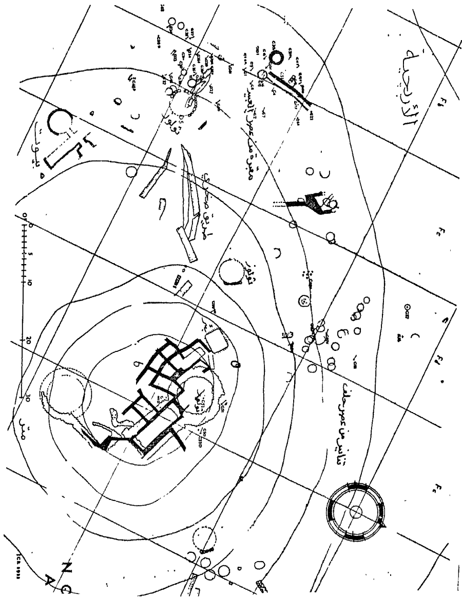
شكل - ٤٦ مخطط تفصيلي يوضح المعالم الرئيسية المكتشفة في تل الاربعية ومنها بقايا الدور
