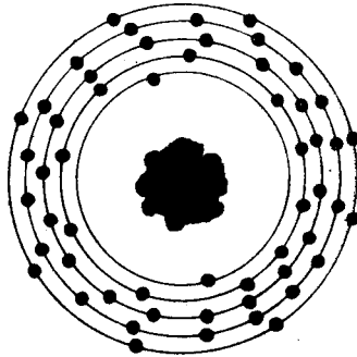
نموذج ذرة
