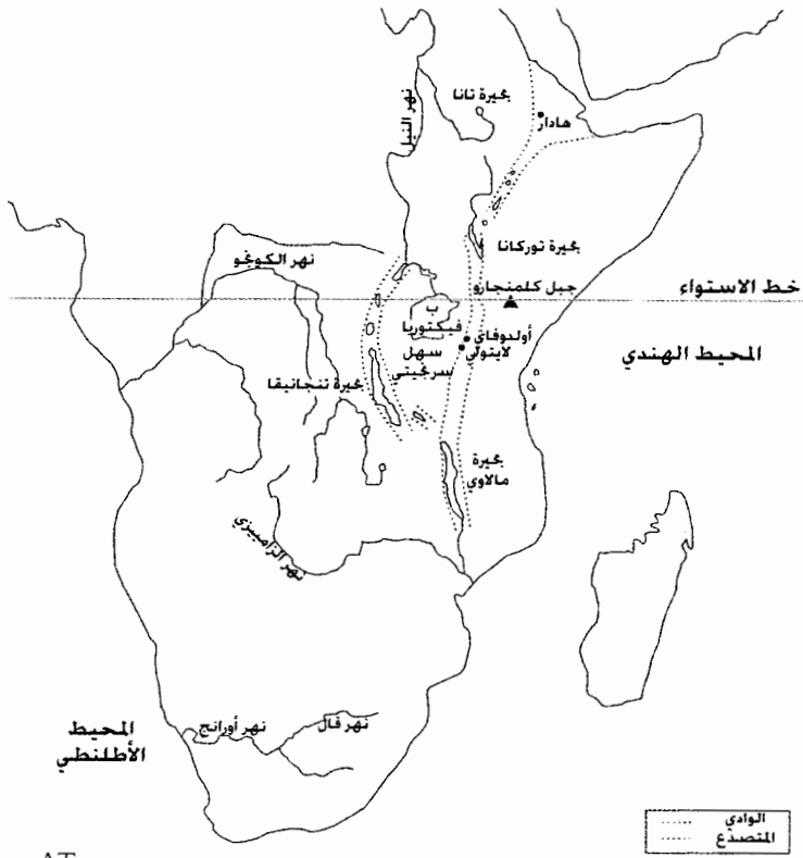
(شكل ٣-٢) الوادي المتصدع الكبير في شرق إفريقيا
