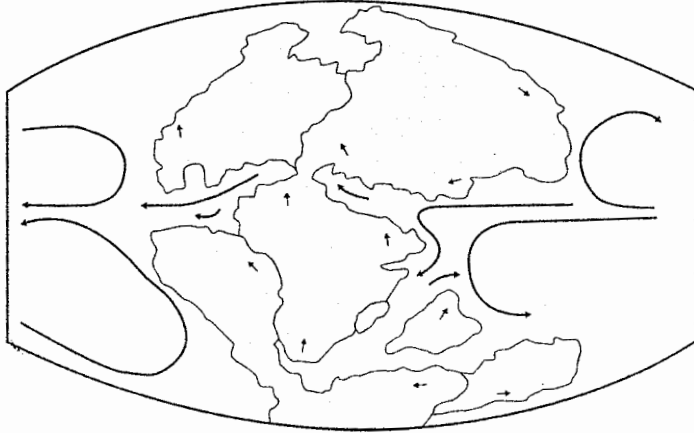
(شكل ٢-٣) تفتت بانجيا منذ حوالي ٢٠٠ مليون سنة
