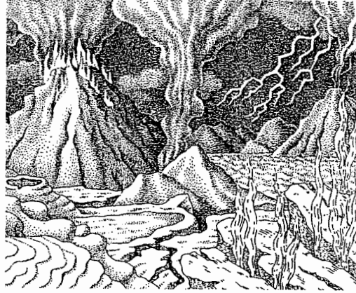
(شكل ٢-١) سطح الأرض منذ حوالي ٤ بليون سنة.
