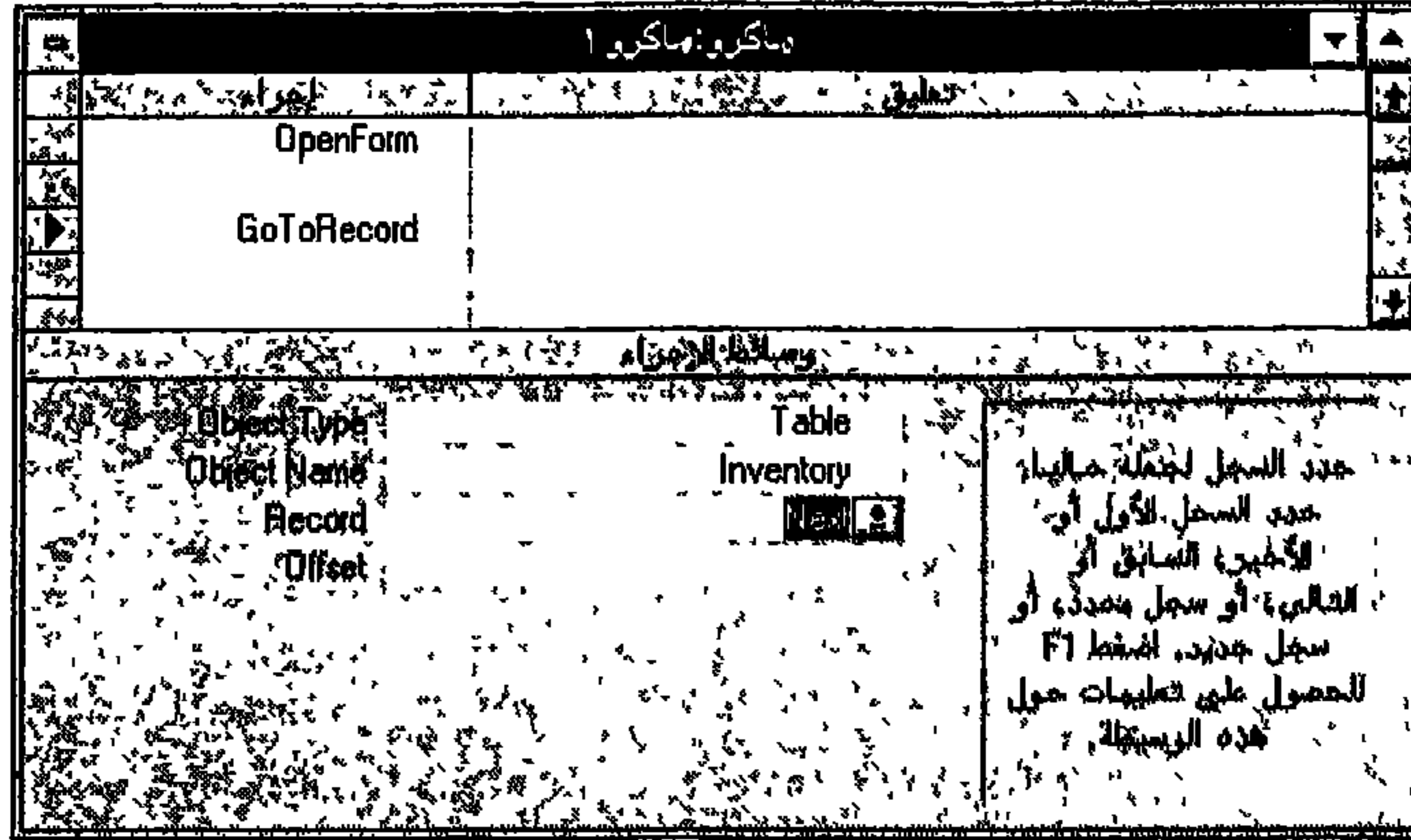
شكل ٣-٧ إجراء GoToRecord
