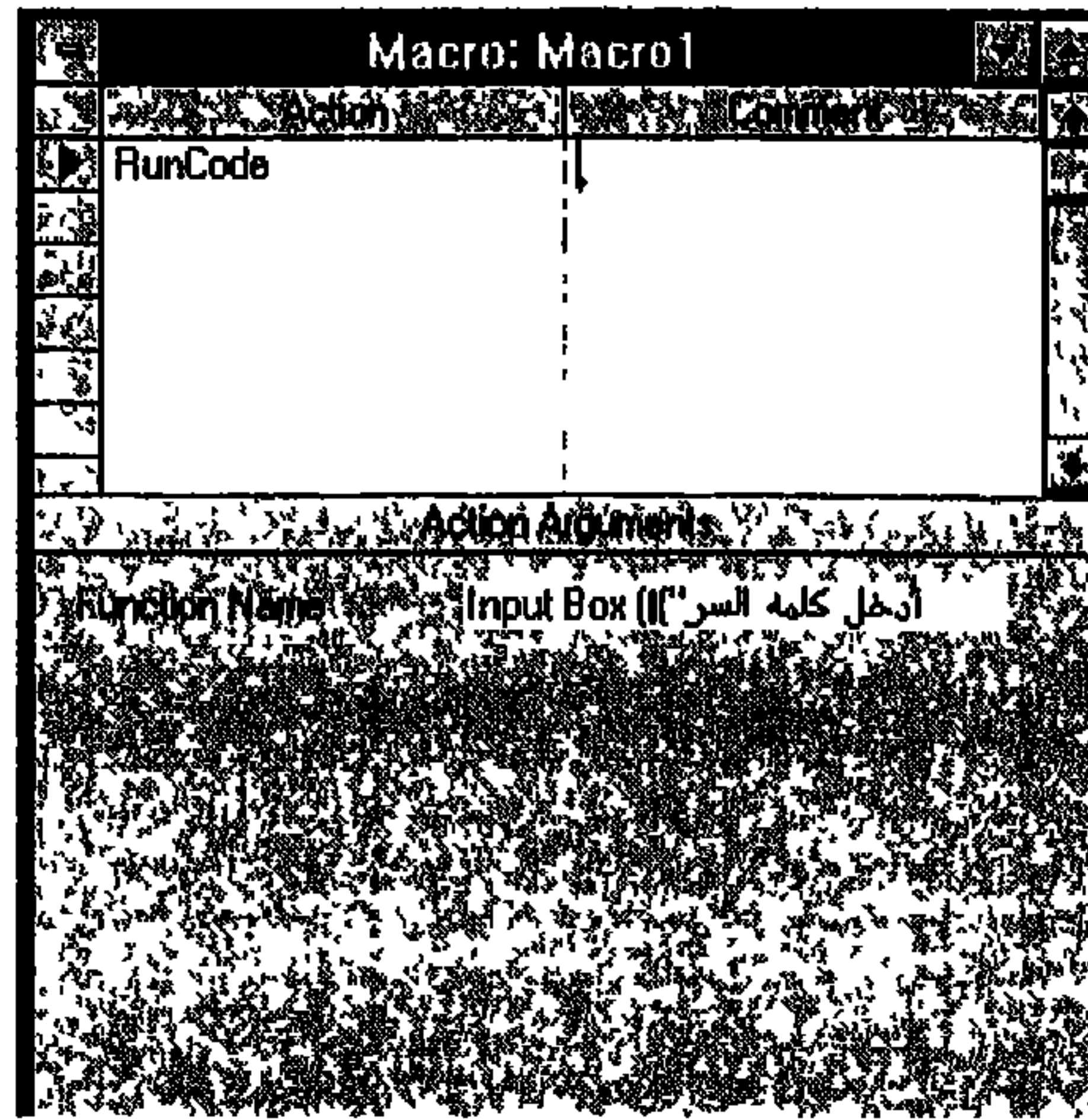
شكل ٢٥-٧ الإجراء RunCode
