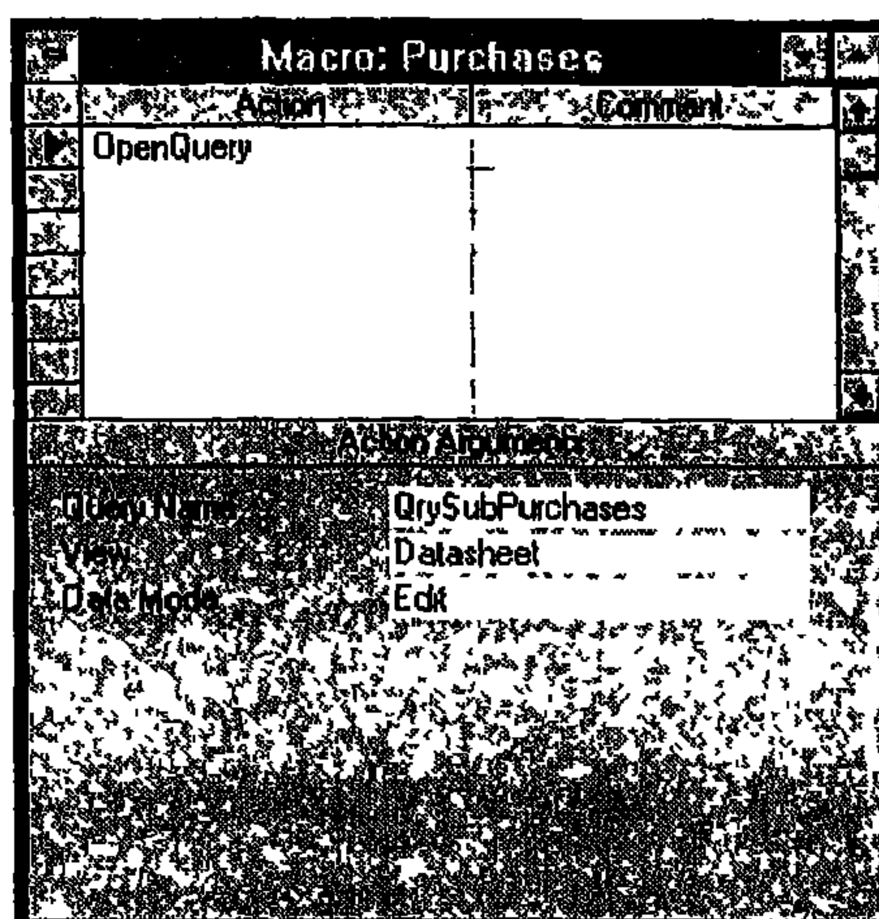
شكل ٧-١٩ إجراء OpenQuery
