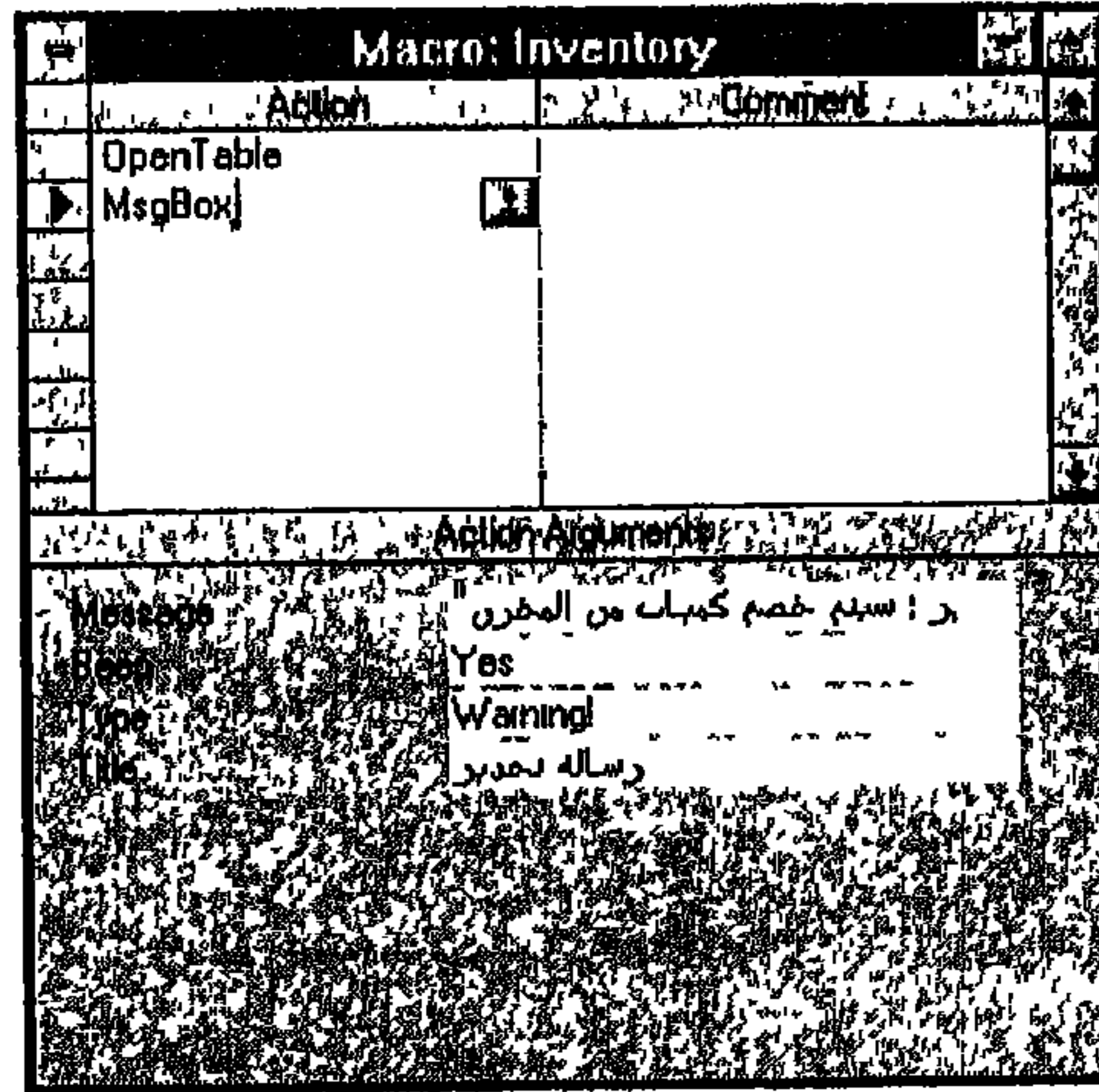
شكل ٧-٢٩ الإجراء MsgBox
