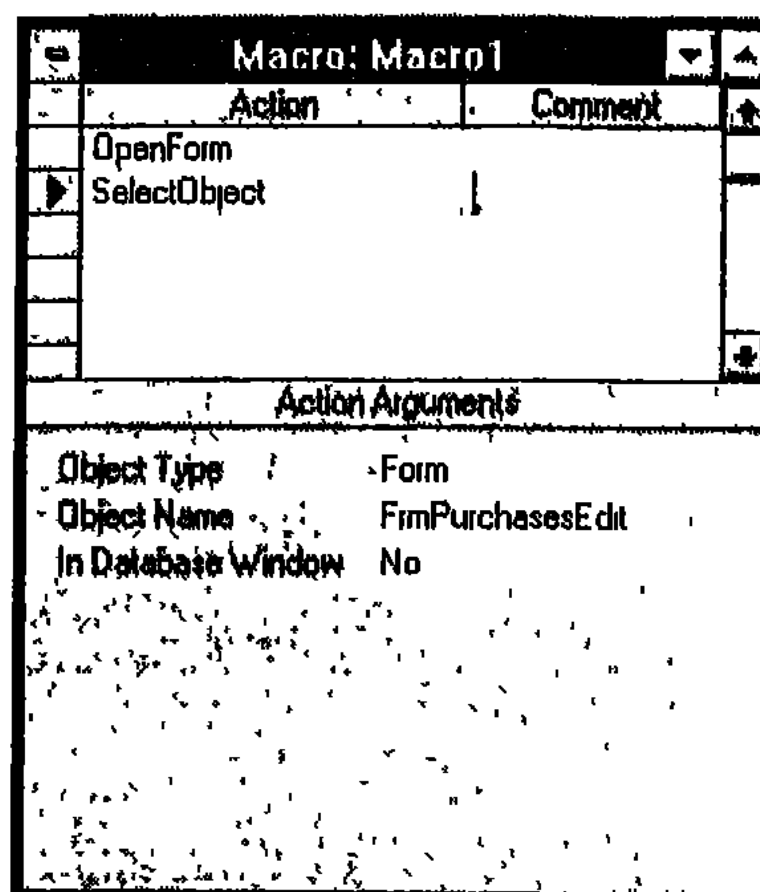
شكل ١٢-٧ الإجراء SelectObject
